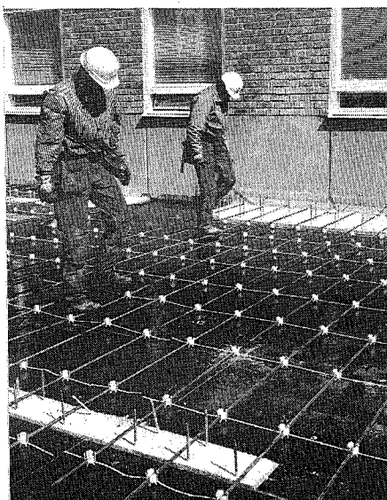
Kloss på band: järnen trampas ner och fixeras i klossarna
